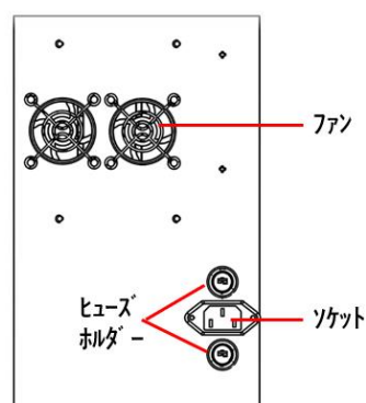
機械背面図
