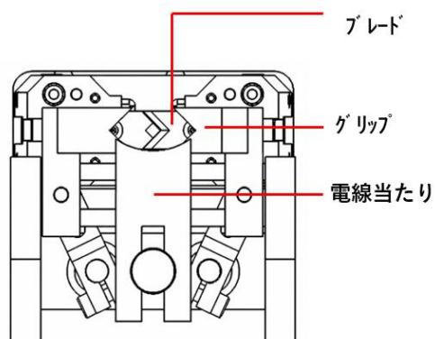
前面機構部
